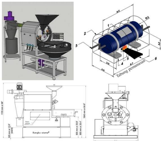
Gambar 1 Desain roaster
